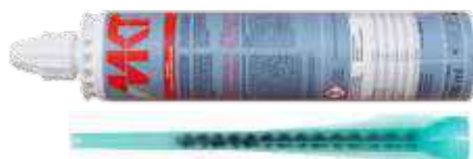
Kartusche VMU plus 300 Schlauchfolien Kartusche für Silikonpistolen geeignet Inhalt: 300 ml
