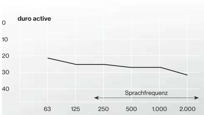
Frequenzabhängige Dämmung
